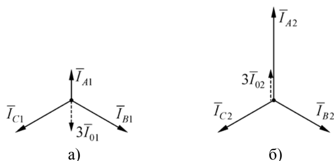
Рис.2. Векторные диаграммы токов в пучке кабелей: а – для верхнего кабеля 1; б – для нижнего кабеля 2
