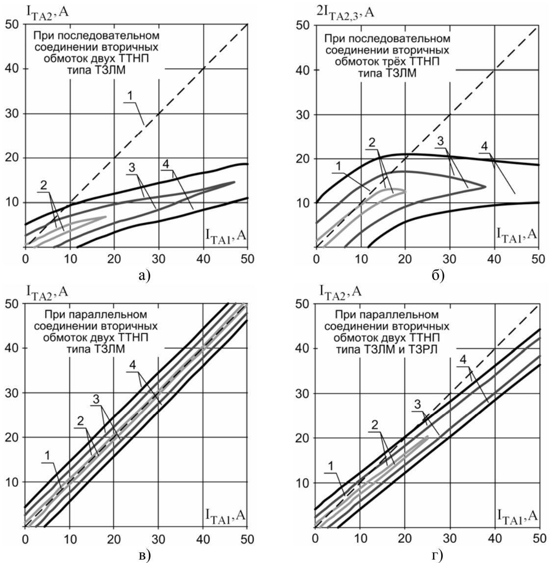
Рис.3. Характеристики срабатывания защиты при нарушении контактных соединений фаз кабелей в пучке:
